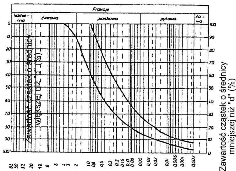
Rysunek 1. Obszar uziarnienia optymalnej mieszanki gliniasto-piaskowej
